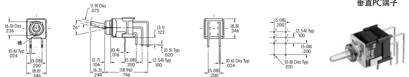
垂直PC端子
