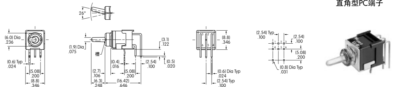
直角型PC端子
